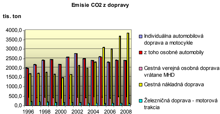
Graf 10 Emisie CO 2 s príspevkom jednotlivých druhov dopravy
